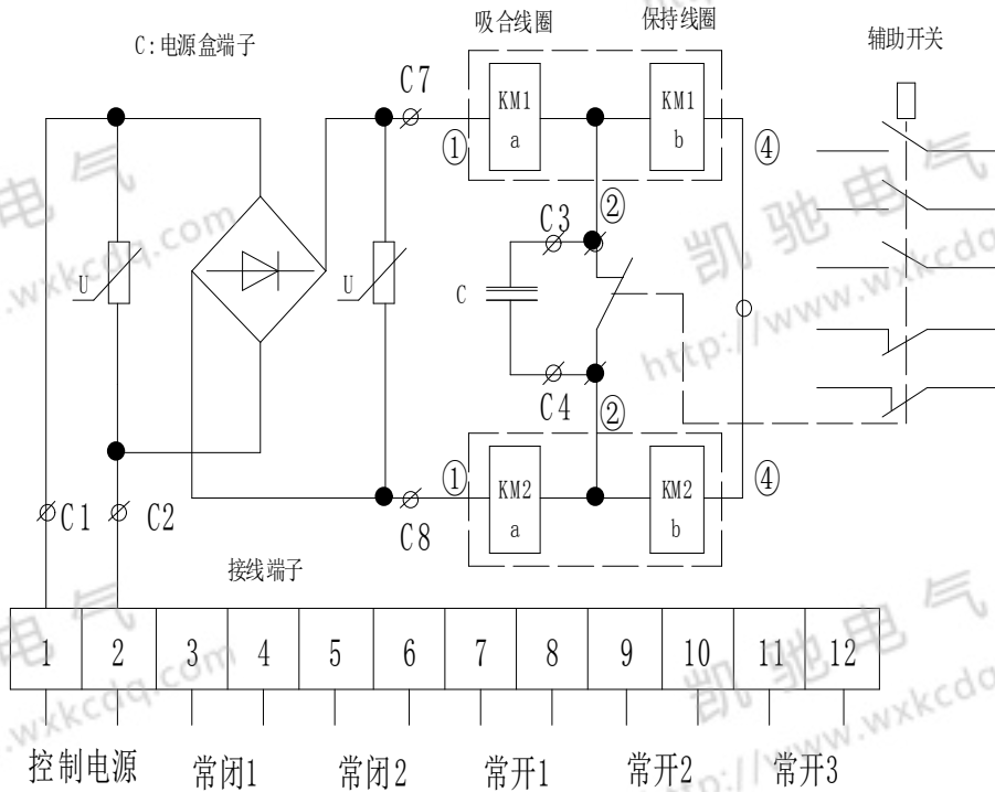
交直流二用电原理及外接线图
