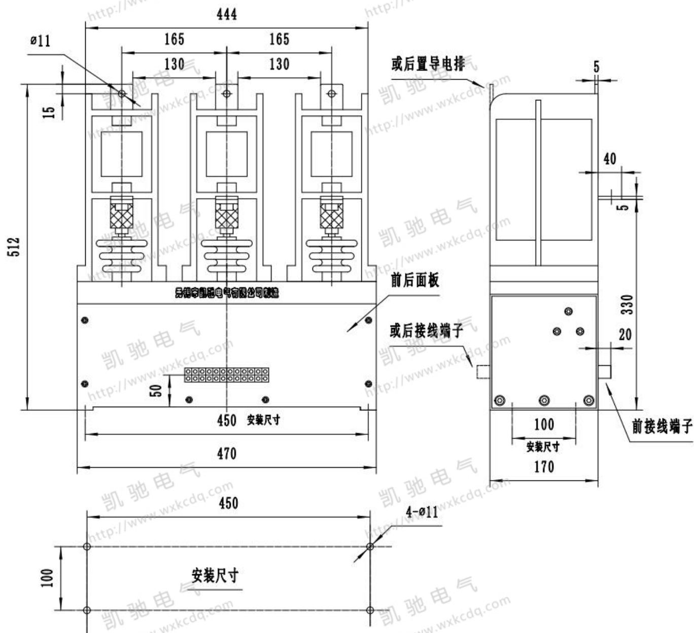
外形及安装尺寸图
